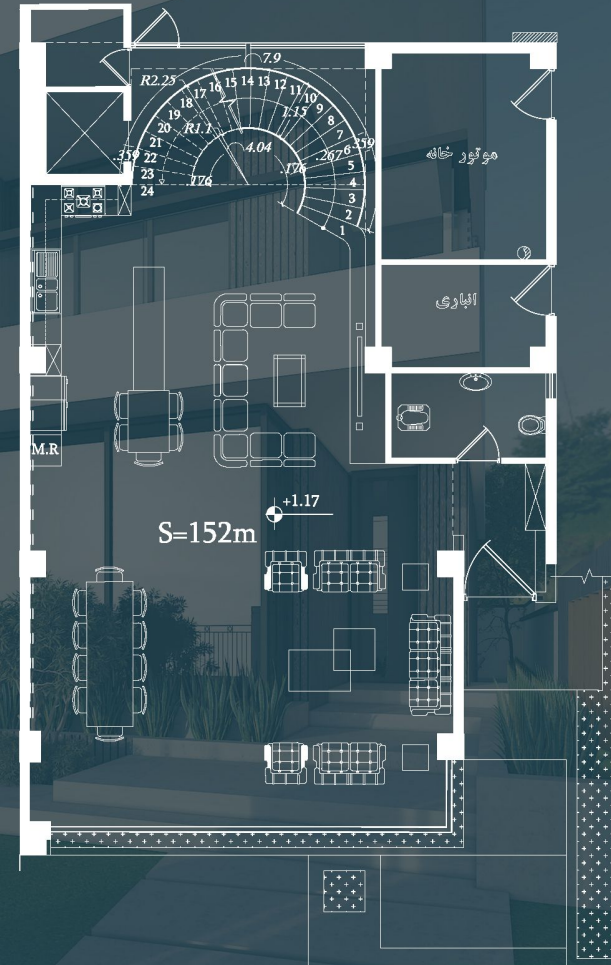
■ پلان طبقه همکف
